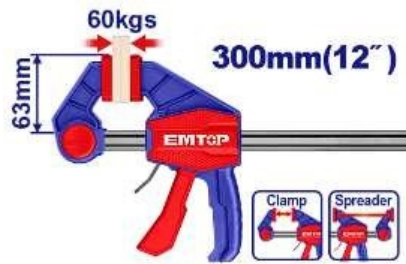
Prensas Barra Rápida 12 - 60 kg EMTOP - ECLPQ60201
