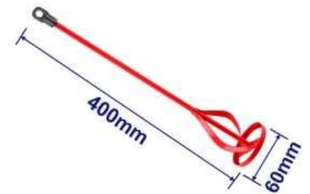
Paleta de mezcla EMTOP - EMXE2306 Longitud: 400 mm Diámetro: 60 mm Grosor: 8 mm Acoplamiento de la herramienta: Hexagonal Orificio de goma para colgar
