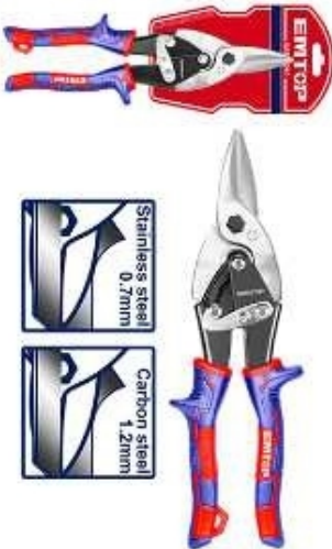
Tijera de Chapa 10" Recta ( 250 mm ) EMTOP - EASP1041 Mango suave de dos tonos de diseño único Tijeras de aviación (rectas) Longitud: 250 mm (10 ") Grosor máximo de corte: Acero al carbono \leq 1,2 mm Acero inoxidable \leq 0,7 mm Envasado en medio blister doble
